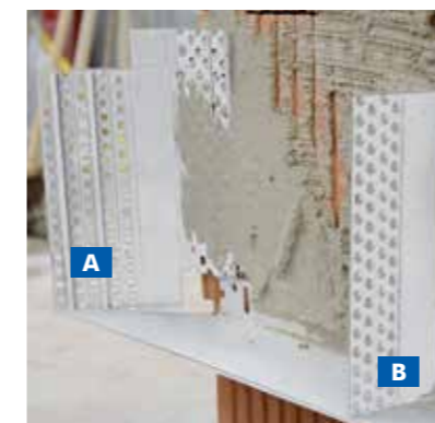
A: maxit eco Eckprofil + Aufsteckprofil klein/groß B: maxit eco Abzugsleiste + Aufsteckprofil klein/groß
